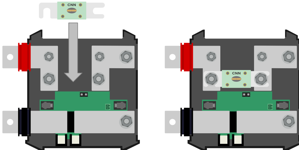
Placera CNN-säkringen i Lynx Shunt VE.Can.
