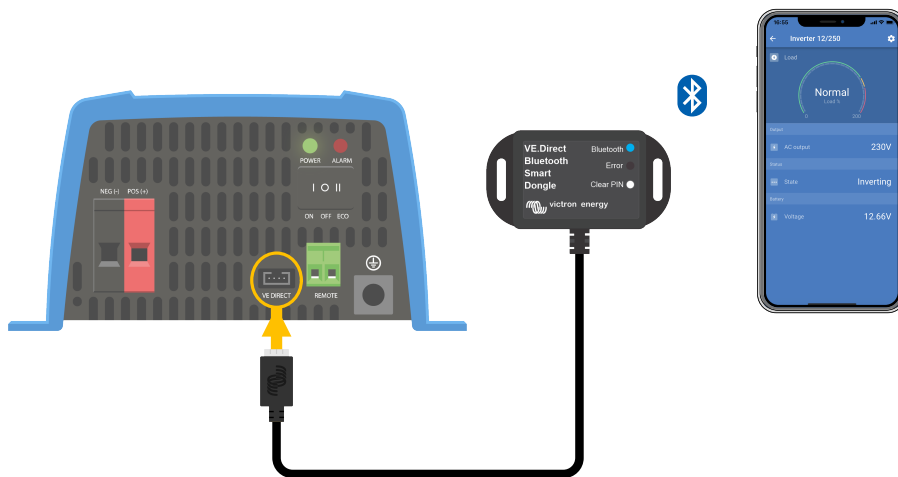
Kopplingschema för VE.Direct Bluetooth Smart-dongle.
